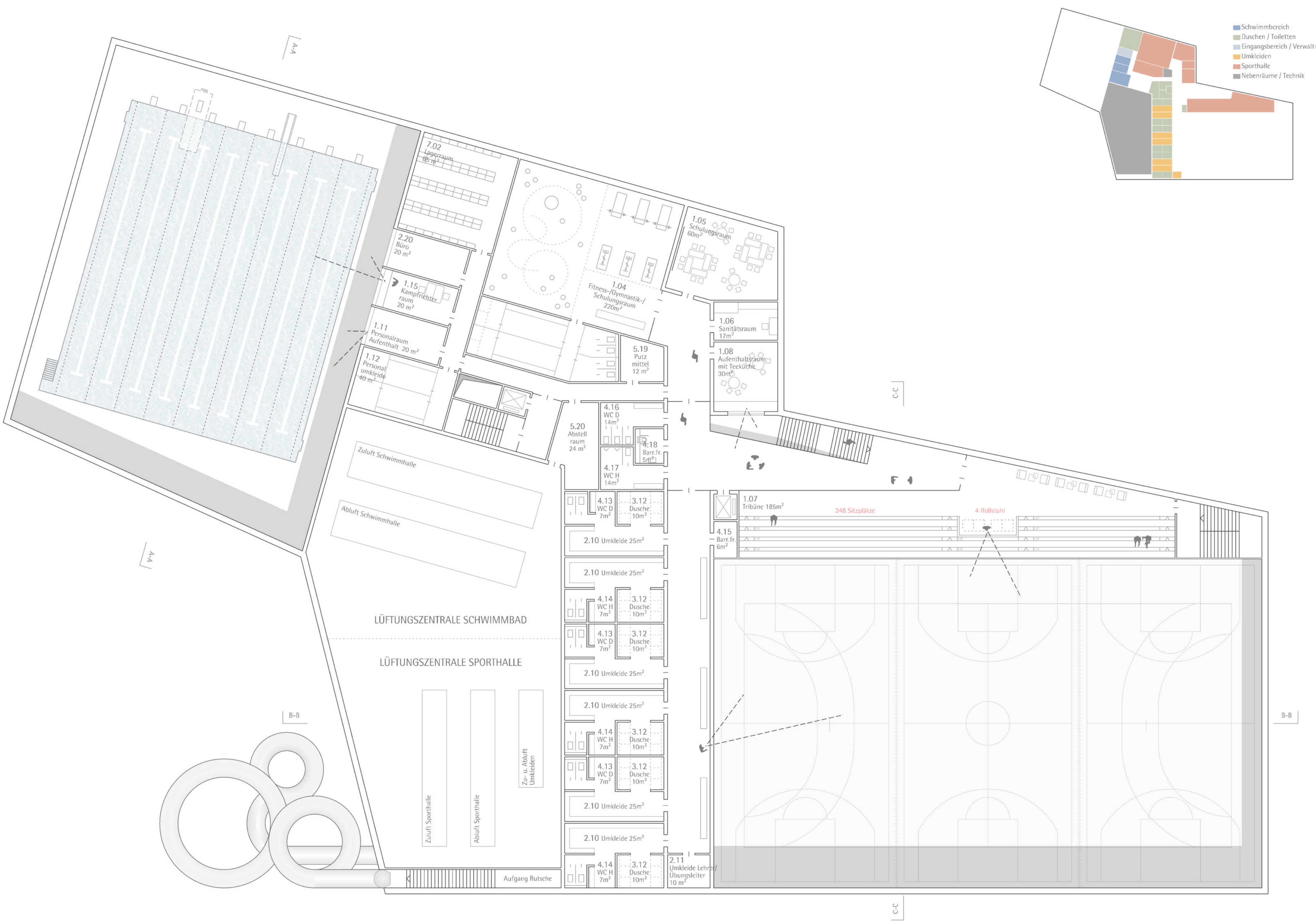
GRUNDRISS OBERGESCHOSS 1:200
