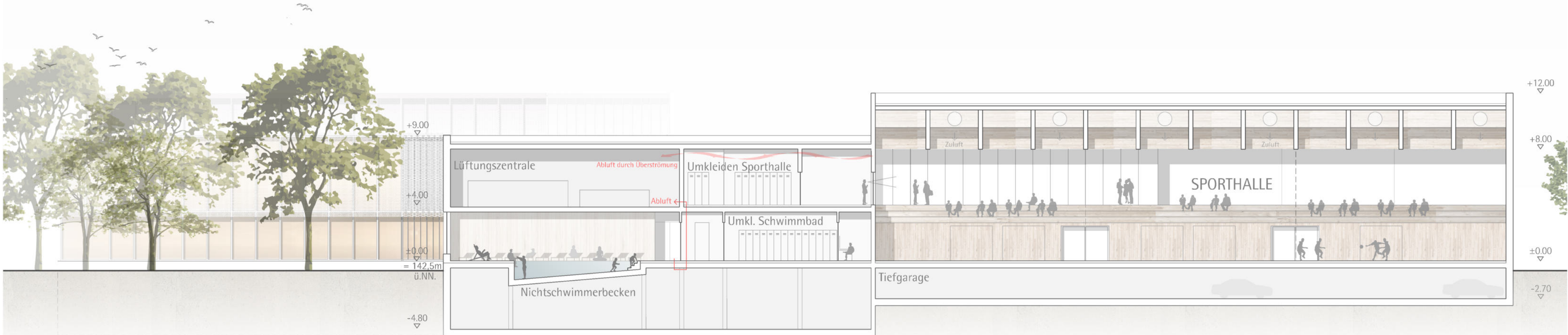
SCHNITT B - B M 1:200
