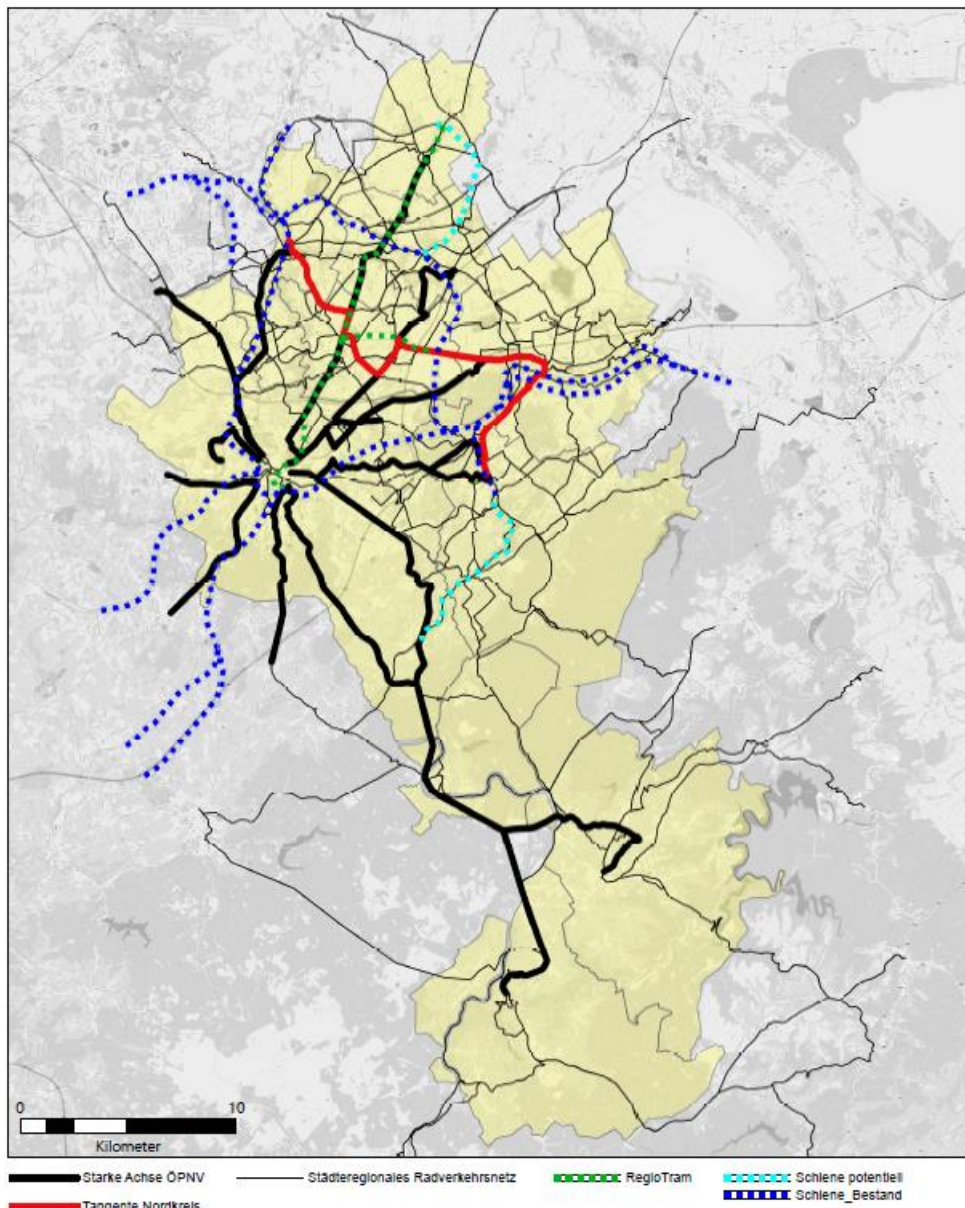
Abbildung 12: Überlagerter Plan AG Starke Achsen/AG Radinfrastruktur inkl. Bestandsschiene (Arbeitsstand: Dezember 2022)
