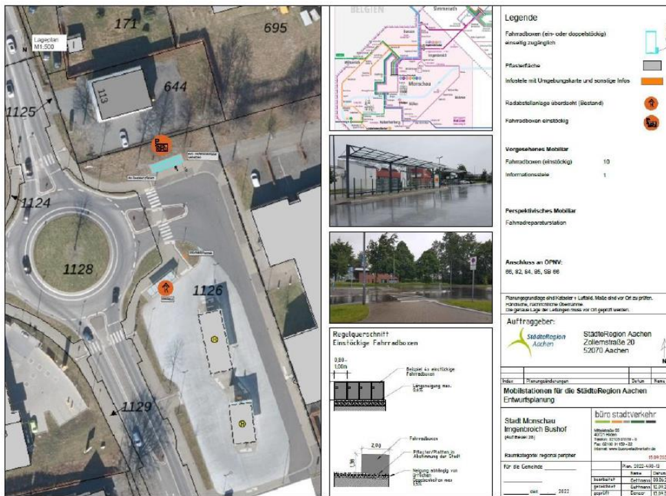
Abbildung 16: Entwurfsplanung Mobilstationen am Beispiel Imgenbroich Bushof
